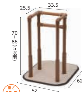
コーナータイプ マット付 PJ01-CSM1 (N)
